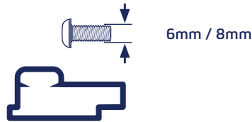
M6 / M8 INSERT
